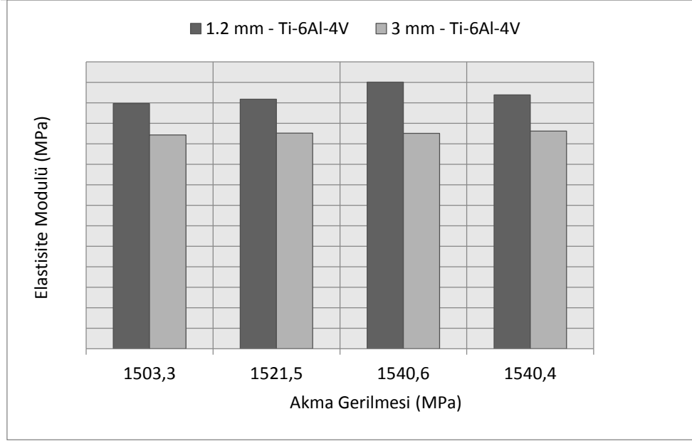
Şekil 7. Elastikiyet Modülü - Akma Gerilmesi Değişimi
