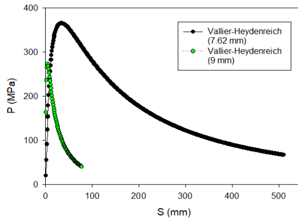
Şekil 7: Basınç Konum Grafiği
